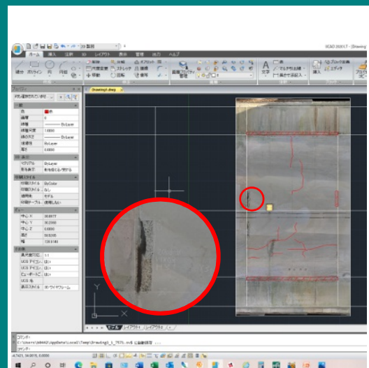
CAD化 自動抽出
